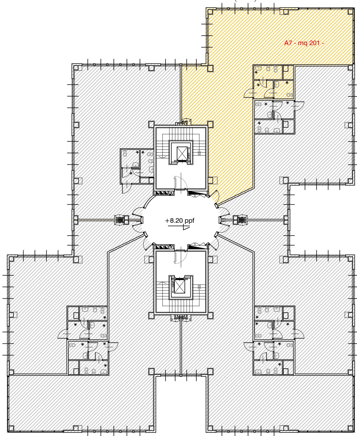
PLANIMETRIA PIANO SECONDO:
